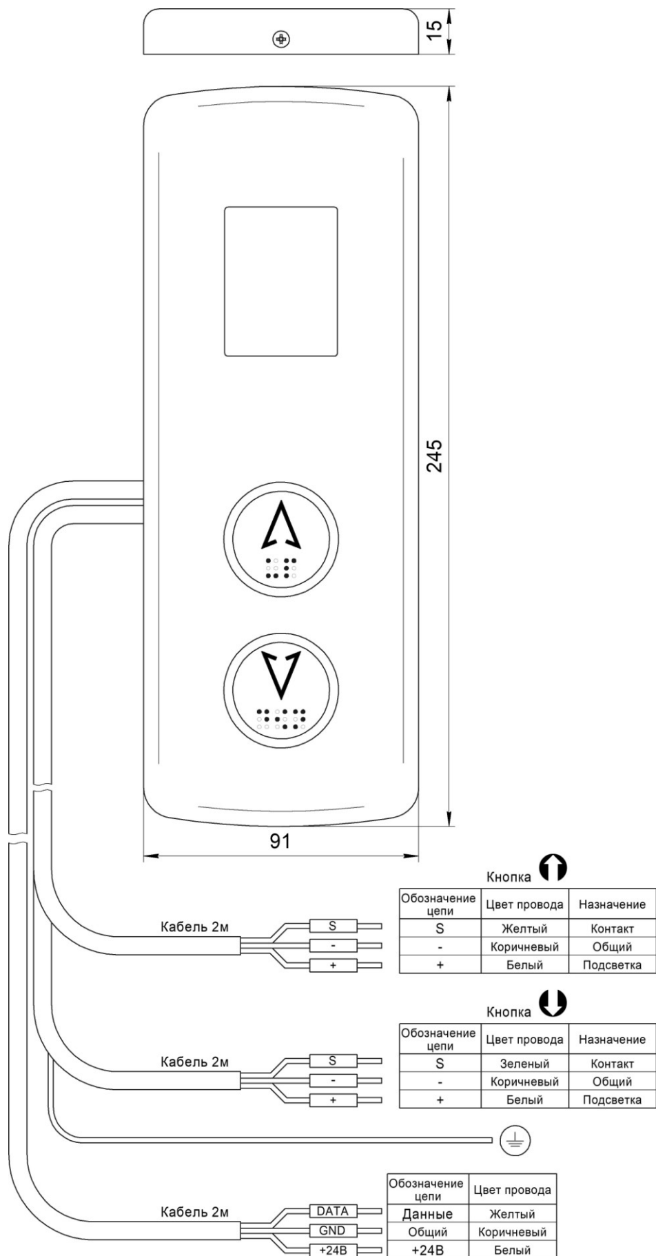
Рис.1 Внешний вид, габаритные и установочные размеры Вызывного поста ЦИРКОН НШЕК.468381.079
